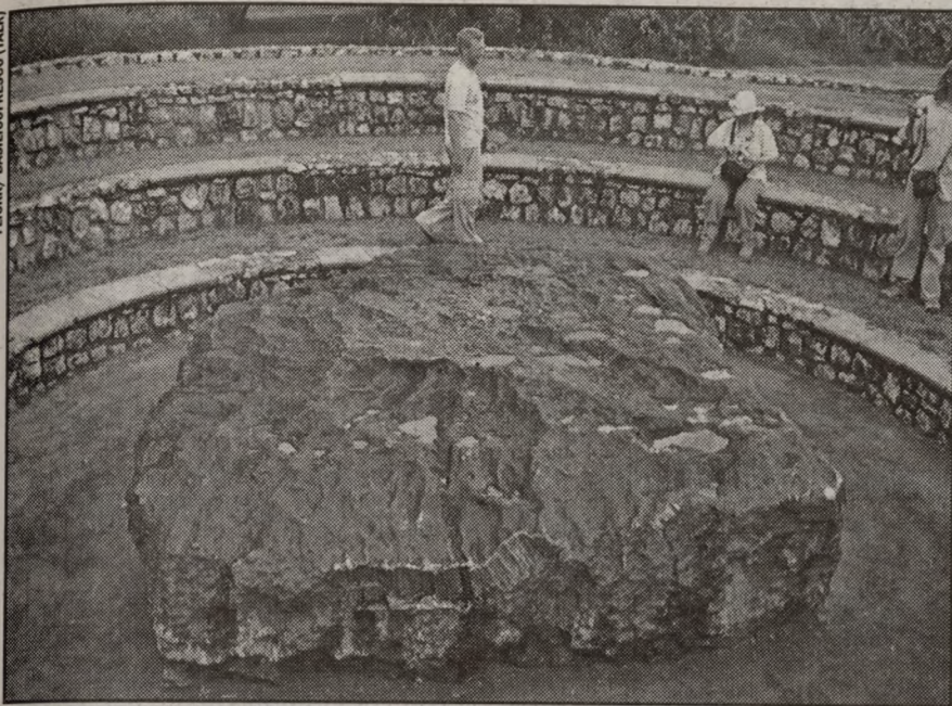
El meteorito Hoba es el más pesado y la masa natural de hierro más grande que se conozca. Fue descubierto en 1920 en la granja Hoba Oeste, cerca de Grootfontein, Namibia. No ha sido movido desde que impactó hace 80 mil años.
